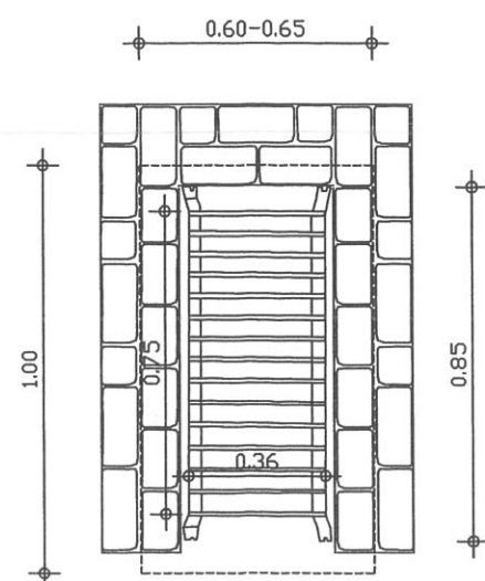
ΚΑΤΟΨΗ
