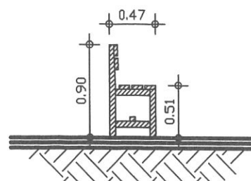
ΤΟΜΗ α-α
