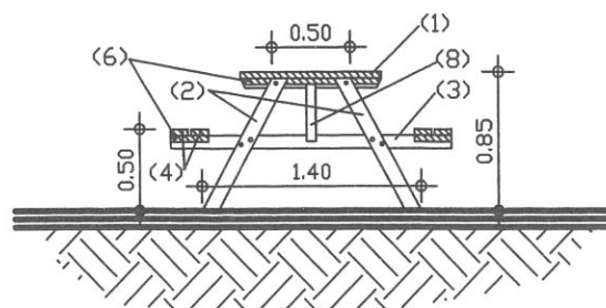
ΤΟΜΗ α-α
